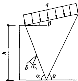
图 L.0.1 计算简图
