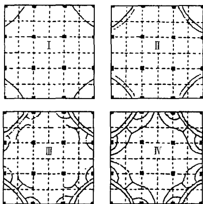
图 37 筏板模型试验裂缝发展过程
