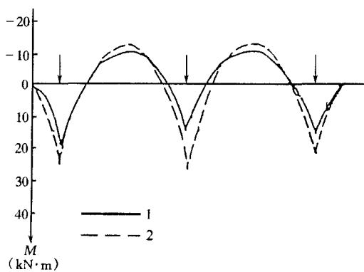
图 42 整体分析法与倒梁板法弯矩计算结果比较
