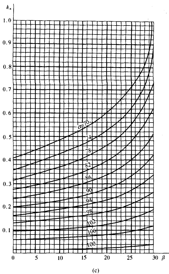
图 L. 0. 2-3 挡土墙主动土压力系数 k_a (三)
