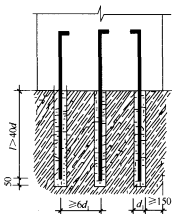
图 8.6.1 锚杆基础
