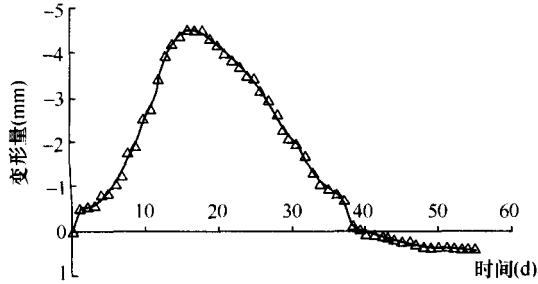
图 17 3 号刚性变形深标点变形时程曲线
