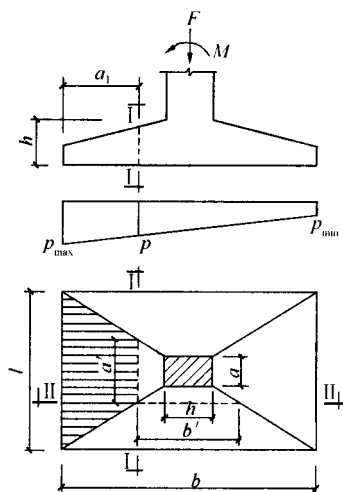
图 8.2.11 矩形基础底板的计算示意
