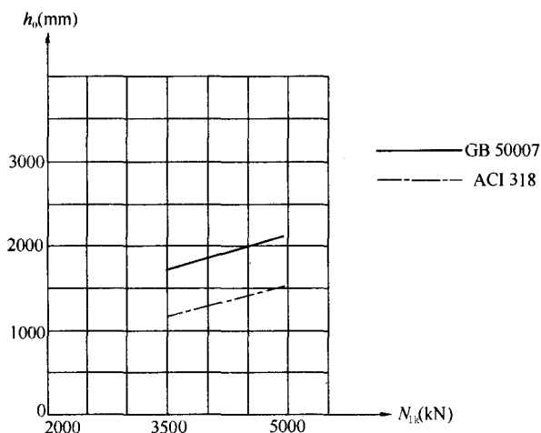
图 51 角桩对承台冲切承台有效高度比较
