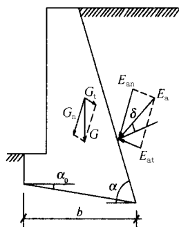
图 6.7.5-1 挡土墙抗滑稳定验算示意
