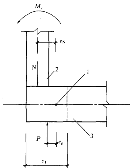
图 33 边柱 M_{\text{unb}} 计算示意
