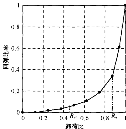
图 13 土样卸荷比—回弹比率、再加荷比—再压缩比率关系曲线（粉质黏土）
