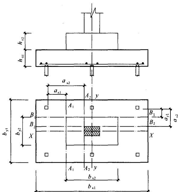
图 U.0.1 阶梯形承台斜截面受剪计算
