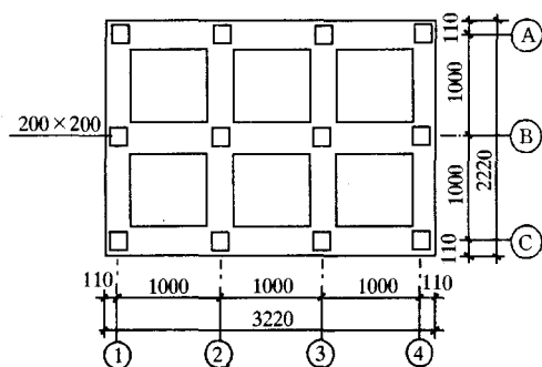
图 39 模型试验加载梁平面图
