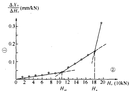
图 S.0.10-2 H_0 - \Delta X_0 / \Delta H_0 曲线
