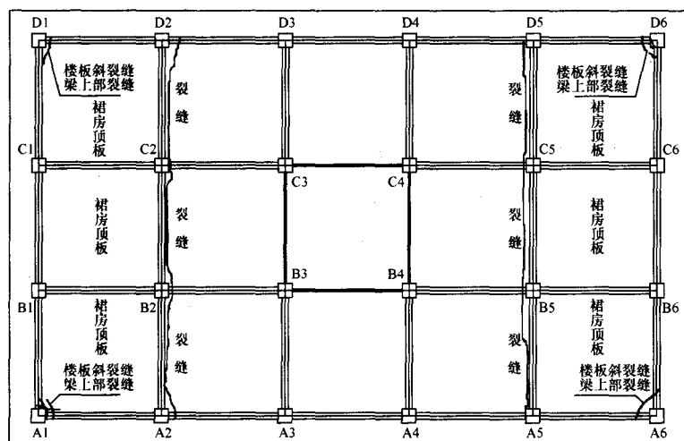
图 48 二层楼板板面裂缝位置图
