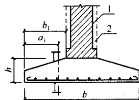
图 8.2.14 墙下条形 基础的计算示意
