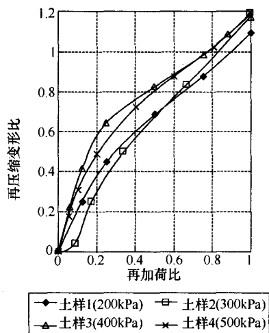
图 18 土工试验所得基底处土体再压缩变形规律
