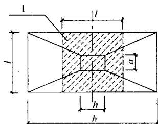
图 8.2.13 基础底板短向 钢筋布置示意
