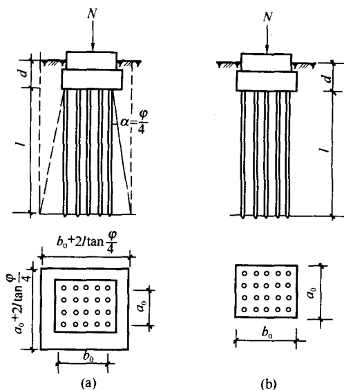
图 R.0.3 实体深基础的底面积
