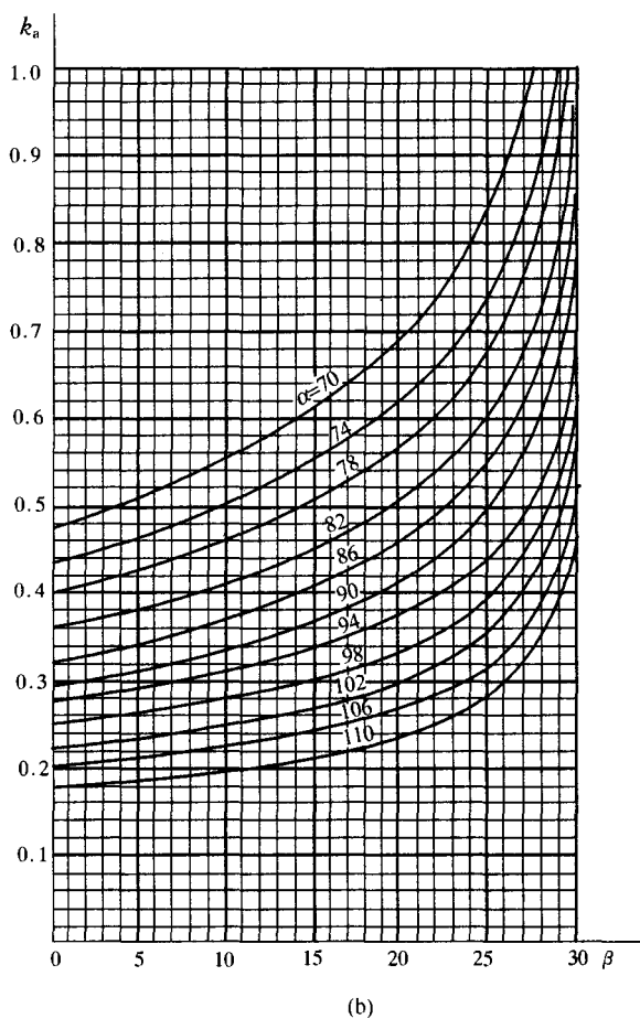
图 1.0.2-2 挡土墙主动土压力系数 k_a (二)
