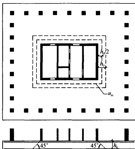
图 8.4.8 筏板受内筒冲切的临界截面位置
