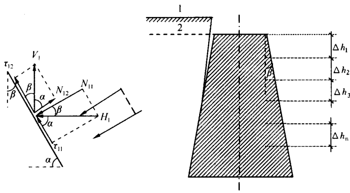
图1 斜面基础基侧受力分布图
