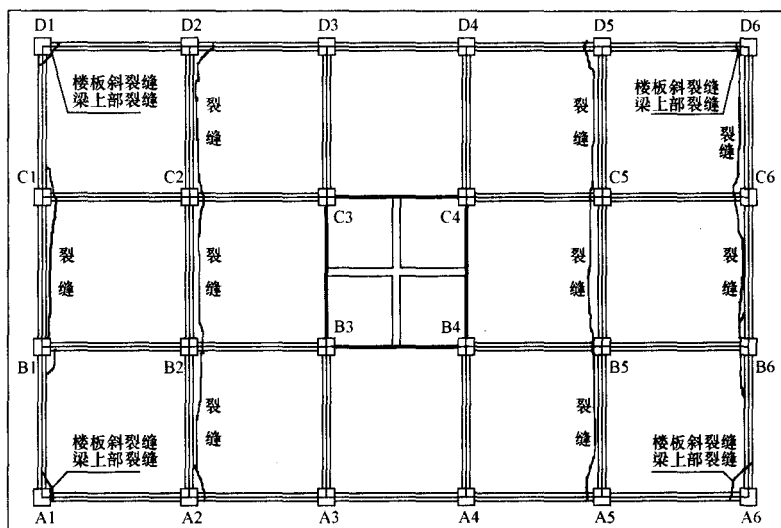
图 47 一层楼板板面裂缝位置图
