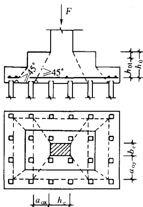
图 8.5.19-1 柱对承台冲切
