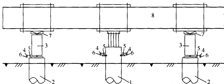
图 T.0.3 单桩竖向抗拔载荷试验示意
