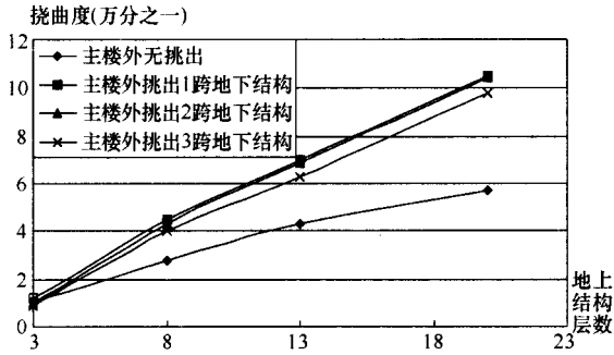
图 22 大底盘高层建筑与单体高层建筑的整体挠曲 （框架结构，2 层地下结构）
