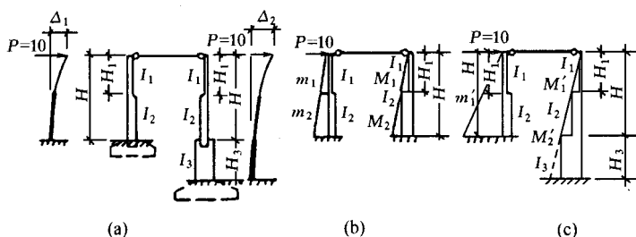
图 29 带短柱基础厂房的计算示意 (a) 厂房图形; (b) 简化计算; (c) 精确计算
