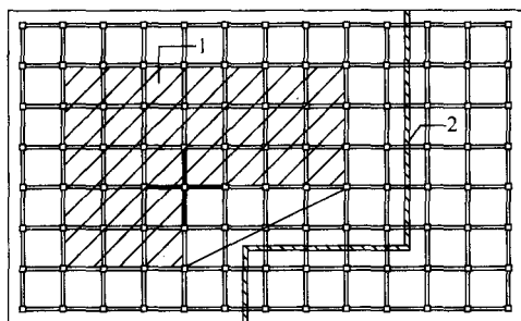
图 44 平面呈 L 形的高层建筑后浇带示意
