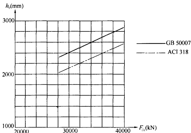
图 50 内柱对承台冲切承台有效高度比较
