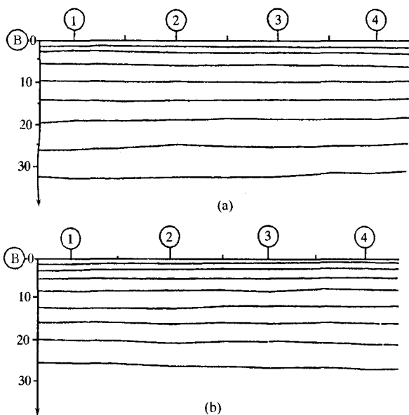
图 41 (B) 轴线沉降曲线
