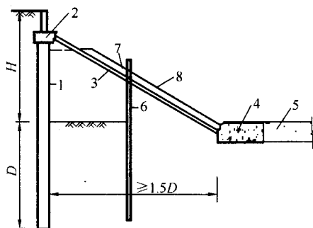
图 57 竖向斜撑体系
