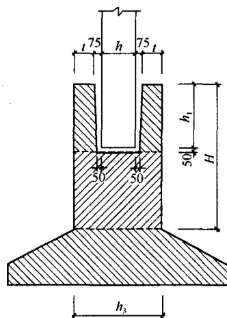
图 8.2.5-1 高杯口基础
