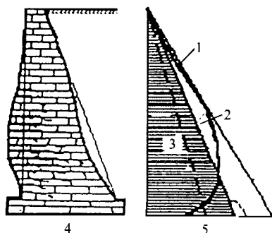
图 24 墙体变形与土压力
