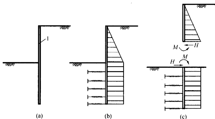
图 55 侧向弹性地基抗力法
