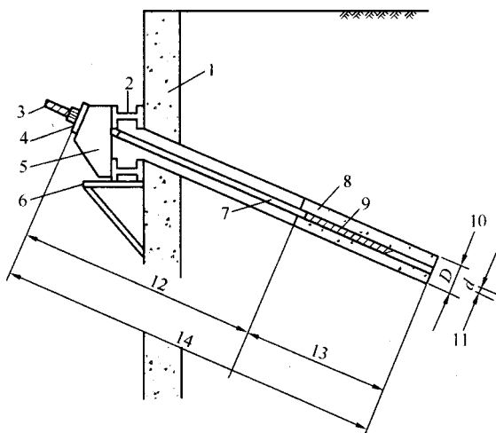
图 59 锚杆构造
