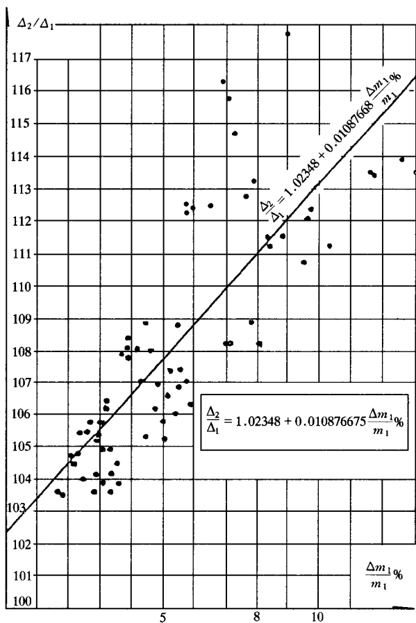
图 30 一般工业厂房 \frac{\Delta_2}{\Delta_1} 与 \frac{\Delta m}{m} \% (上柱) 关系
