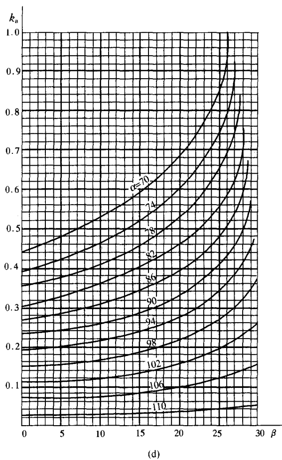
图 L. 0. 2-4 挡土墙主动土压力系数 k_a (四)
