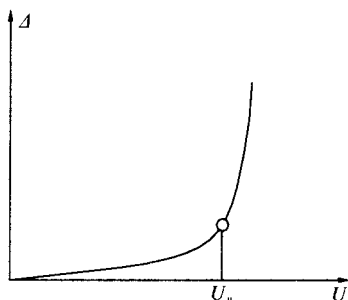
图 T. 0. 10-1 陡变形 U-\Delta 曲线
