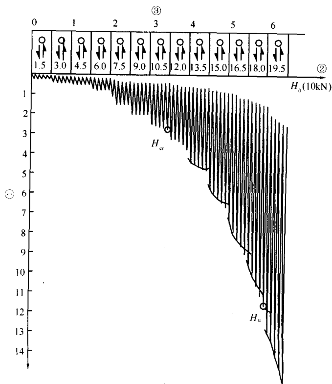
图 S.0.10-1 H_0-t-X_0 曲线
