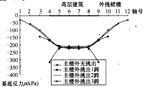
图 23 大底盘高层建筑与单体高层建筑的基底反力 （内筒外框结构 20 层，2 层地下结构）
