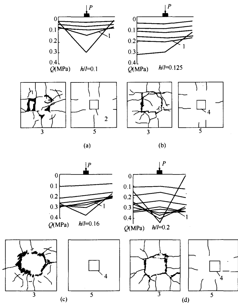
图 31 不同宽高比的基础板下反力分布
