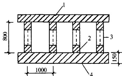
图 40 模型试验 (B) 轴线剖面图
