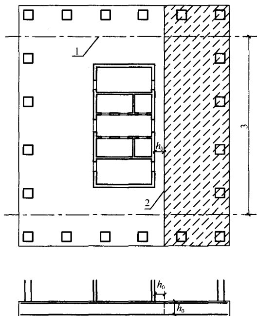
图 38 框架-核心筒下筏板受剪承载力计算截面位置和计算
