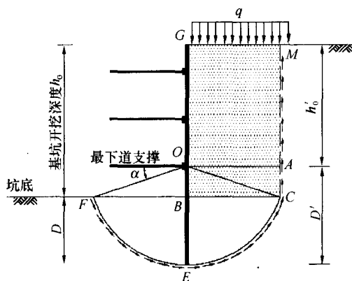
图 56 坑底抗隆起计算简图
