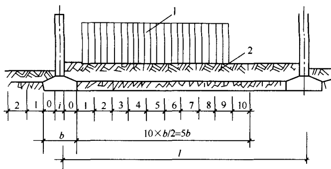
图 N. 0. 4 地面荷载区段划分
