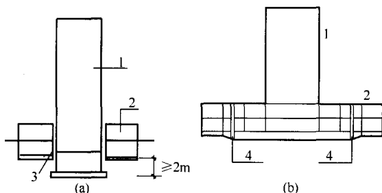
图 8.4.20 高层建筑与裙房间的沉降缝、后浇带处理示意
