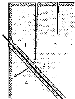
图 6.8.2-1 边坡顶部支护 1—崩塌体; 2—岩石边坡顶部 裂隙; 3—锚杆; 4—破裂面
