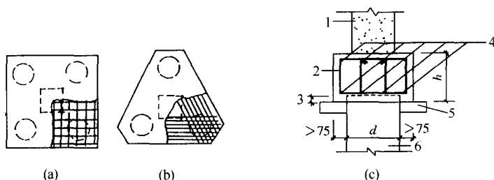
图 8.5.17 承台配筋
