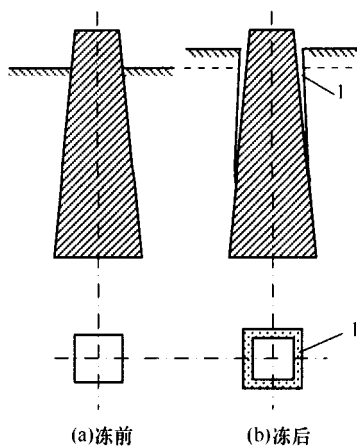
图3 斜面基础的防冻胀试验
